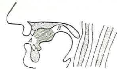
Fig. 28 Vocalele anterioare.
