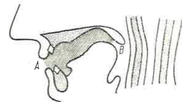
Fig. 30 Vocalele posterioare.
