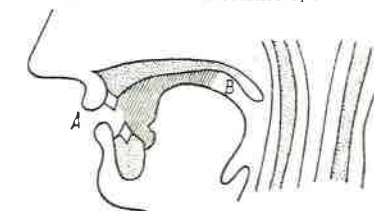
Fig. 29 Vocalele mediale.
